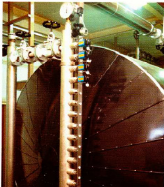
Realisierung von 4 unabhängigen Schaltepunkten mit Liquiphant-Vibrationssonden im Standrohr eines Sammelbehälters für Kesselspeisewasser
