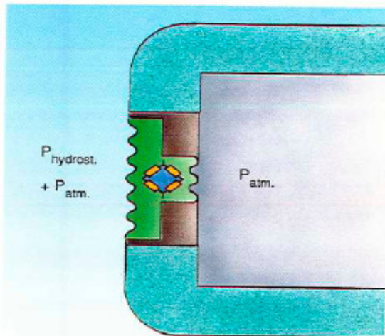
Hermetisch geschlossene Meßzelle
