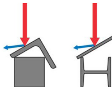
Abb. 6.11: Ein Streublech verteilt die Mikrowellenenergie zur Seite und reduziert damit die Störeoamplitude.
