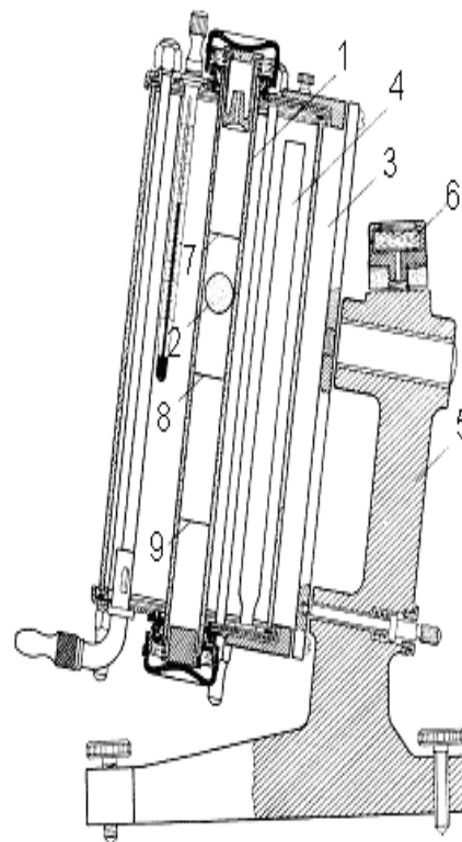
Höppler-Viskosimeter
