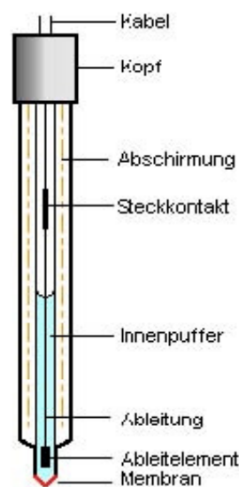
Messelektrode
