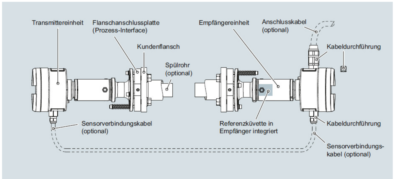
Aufbau des SITRANS SL-Systems in Nicht-Ex-Ausführung
