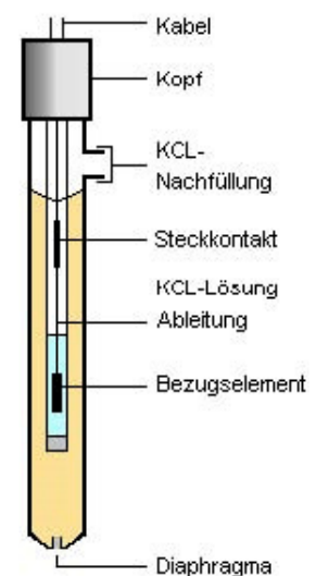
Vergleichselektrode
