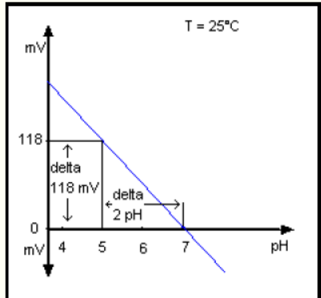
Steilheit
