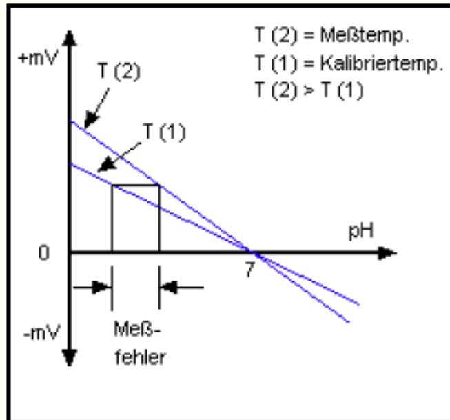
Temperatureinfluss
