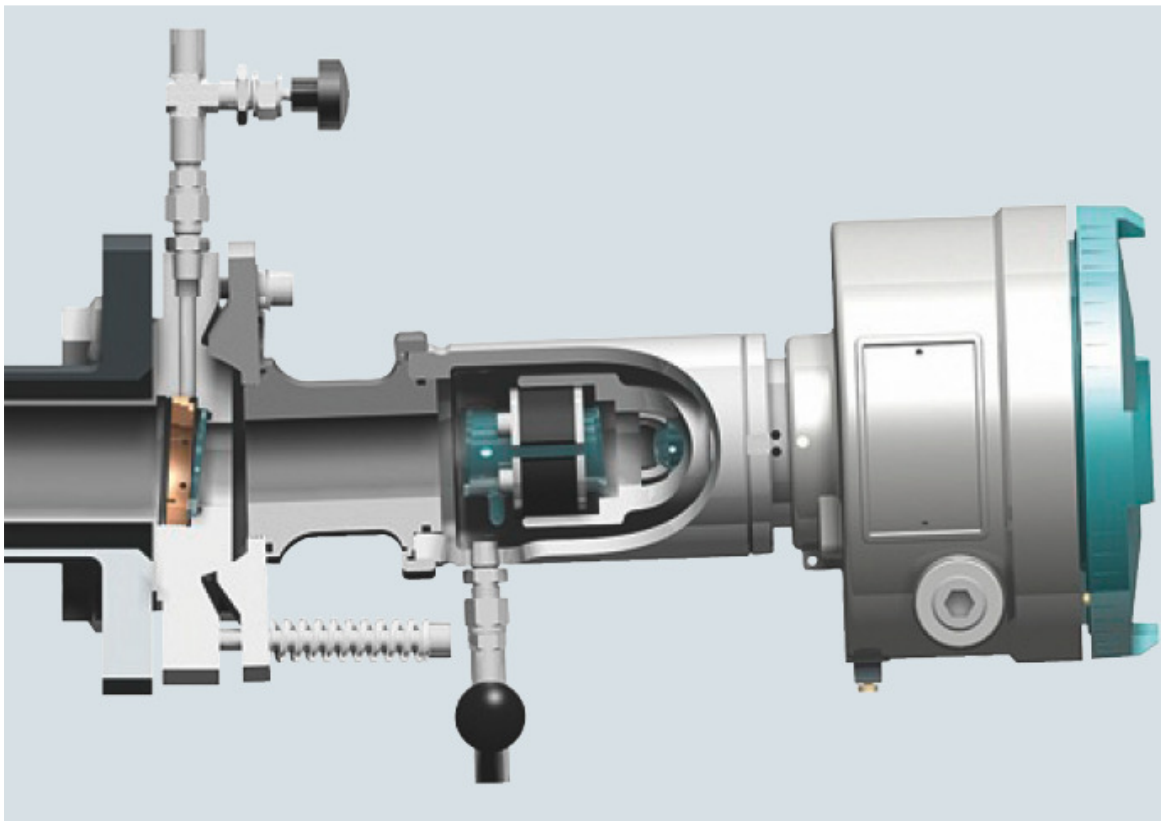
SITRANS SL, Empfängereinheit
