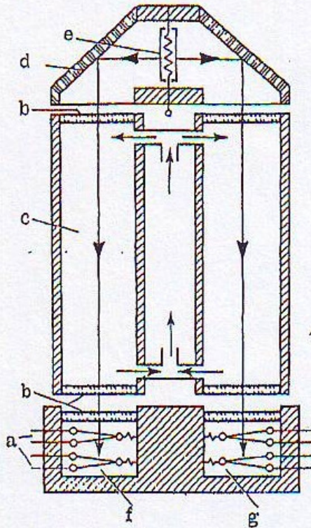
Bild 157 Gasanalyse durch Infrarotabsorption (Siemens)
