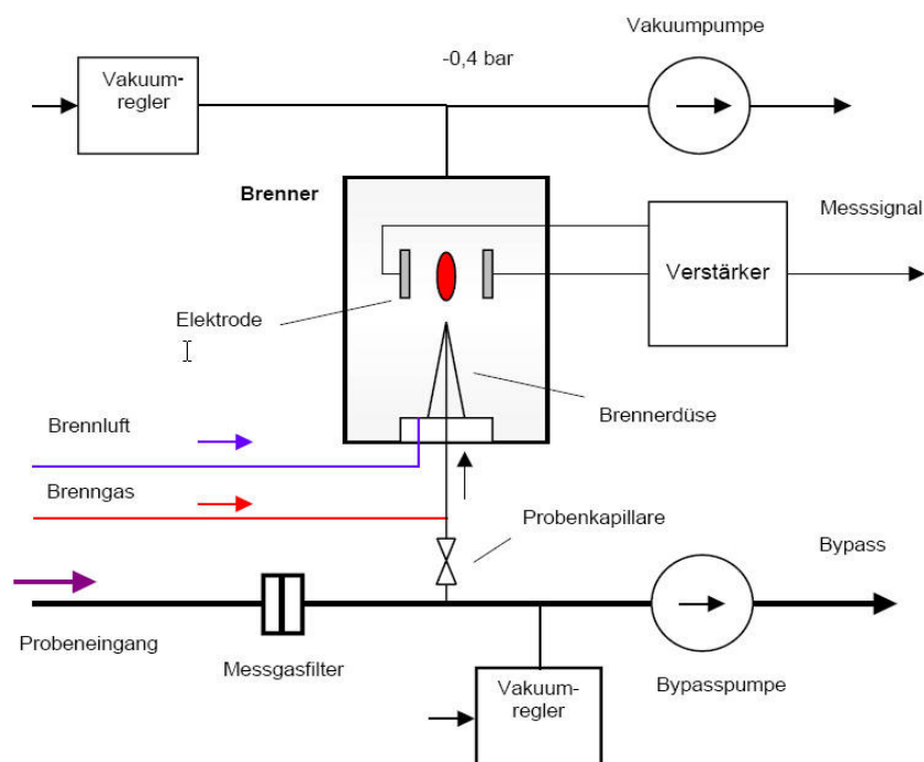
Prinzipdarstellung Flammenionisationsdetektor (Vakuum-FID)
